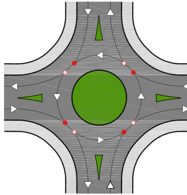
Figura 23. Punts de conflicte en una rotonda
