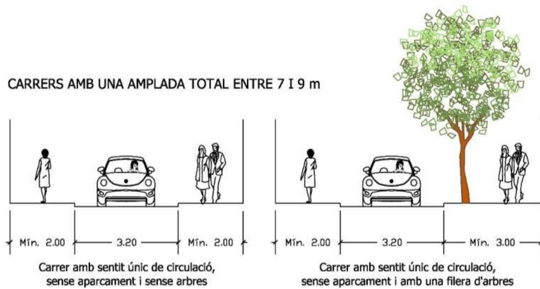
Figura 14. Seccions per a carrers amb amplada de 7 a 9 metres
