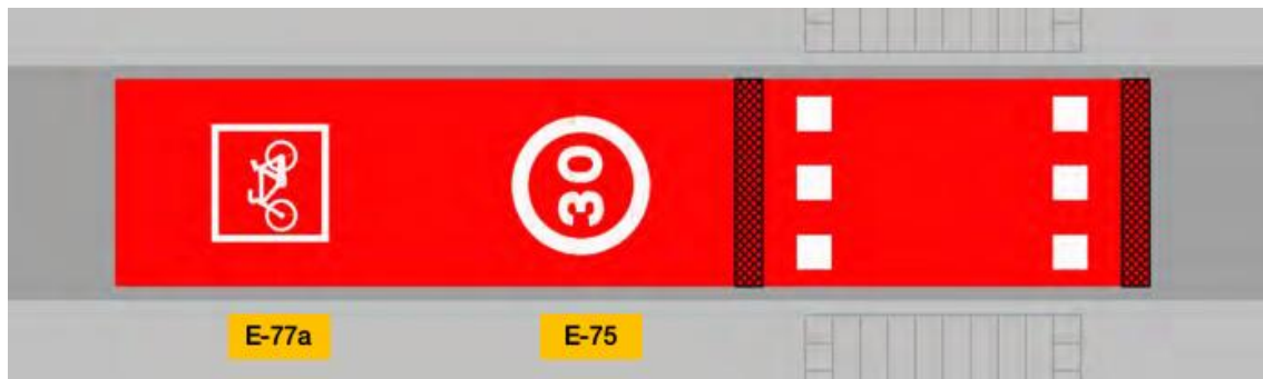
Figura 44. Exemple d'accés a carrer de zona 30: Pas de vianants elevat per reduir la velocitat dels vehicles i senyalització horitzontal
