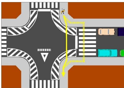
Figura 29. Intersecció igual que l'anterior, amb marques viàries de zona morta
