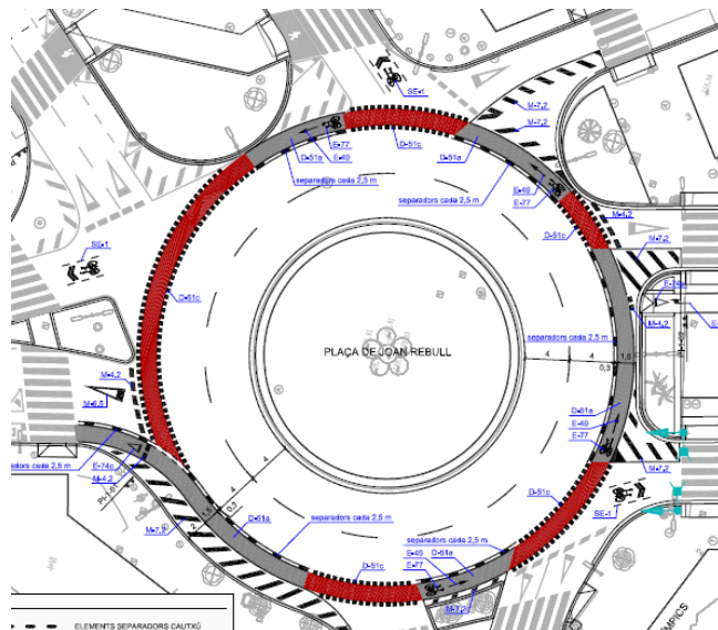
Figura 45. Exemple de configuració de carril pedalable segregat en rotonda
