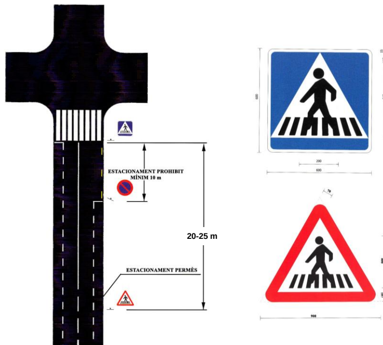
Figura 41. Senyalització vertical d'un pas de vianants
