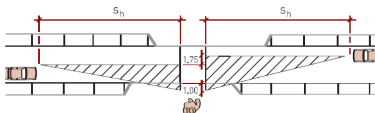
Figura 32. Paràmetres pel càlcul de les distàncies de visibilitat dels vianants
