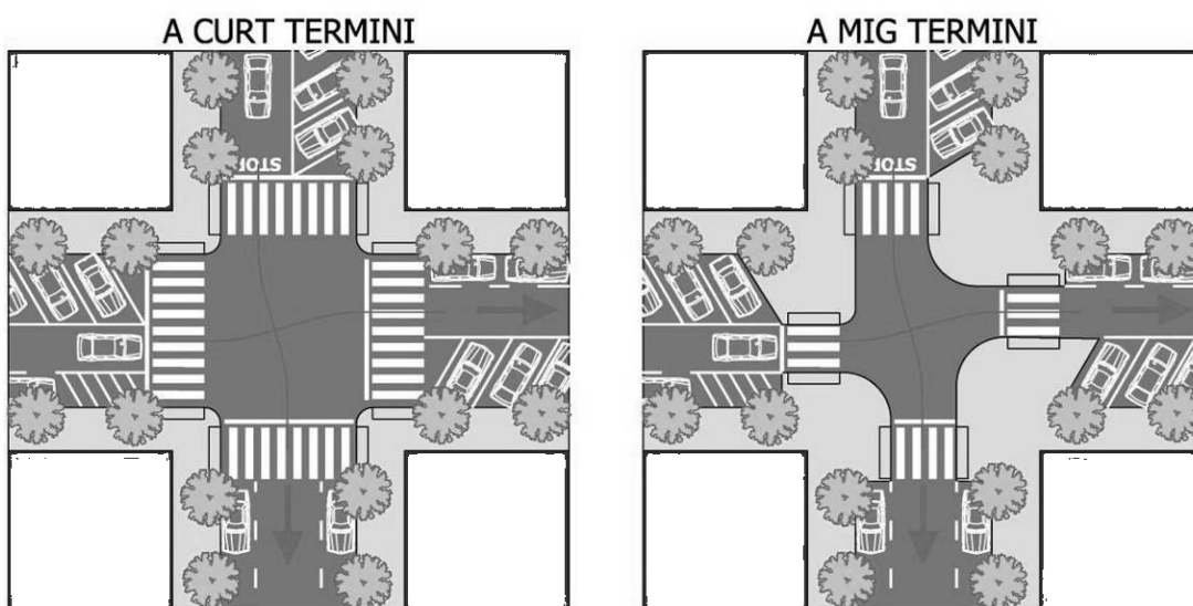
Figura 19. Aplicació de reductors horitzontals de velocitat a carrers amb calçades amples
