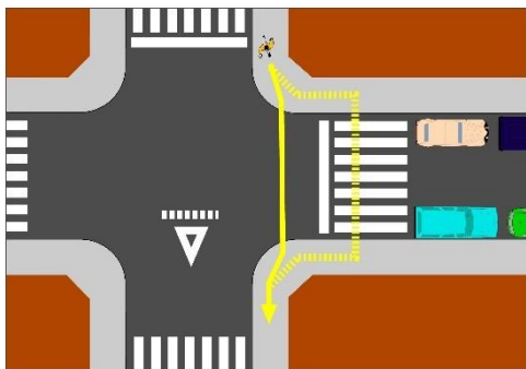
Figura 28. Intersecció no compacta. Pas de vianants fora de la trajectòria idònia del vianant
