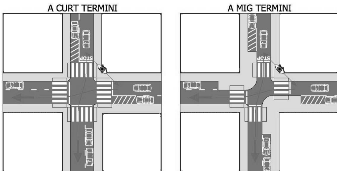
Figura 17. Aparcament alternat de costat per a reduir la velocitat. Solució provisional i solució definitiva
