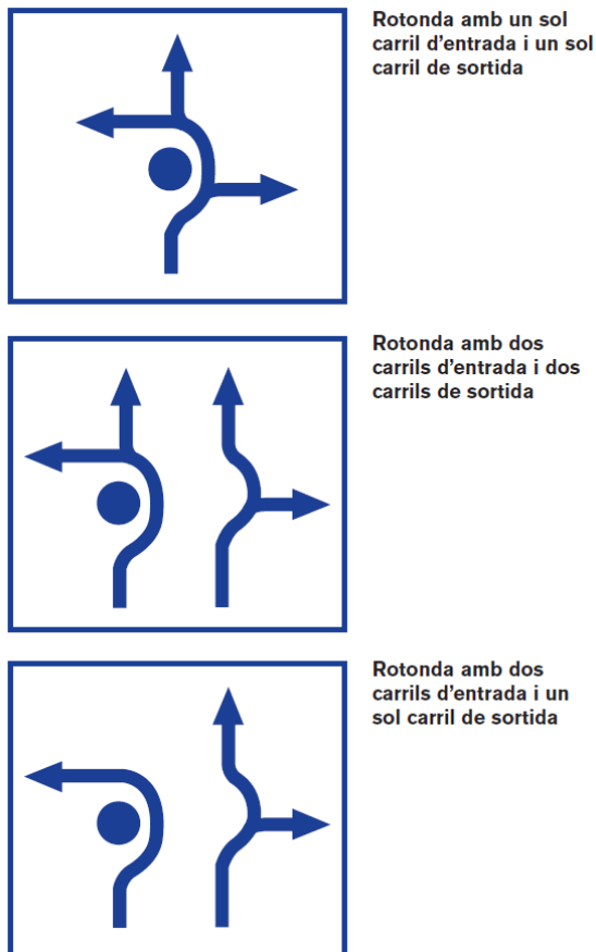
Figura 51. Proposta de fletxes de direcció prèvies a la rotonda
