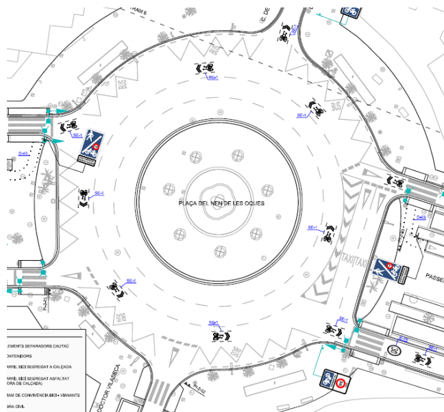
Figura 46. Exemple de configuració de circulació en calçada de bicicletes en rotonda (pictogrames)
