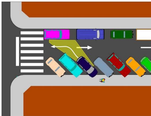
Figura 36. Sortida semibateria amb visibilitat insuficient
