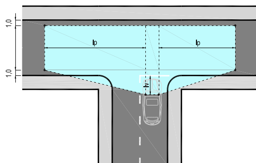
Figura 27. Àrea de visibilitat en interseccions en T
