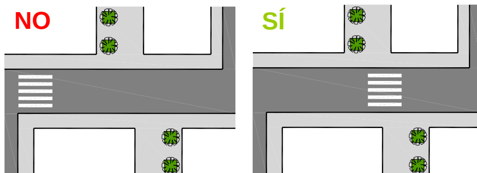
Figura 39. Recomanacions d'ubicació de passos de vianants
