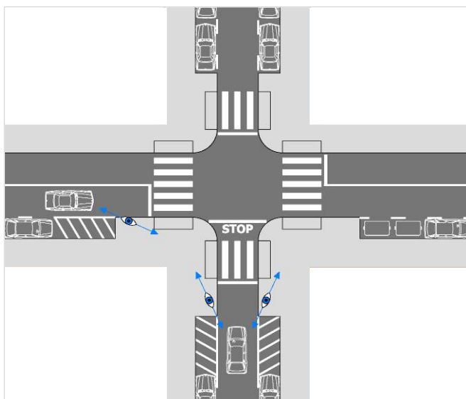
Figura 34. Exemple d'aplicació d'orelles als passos de vianants
