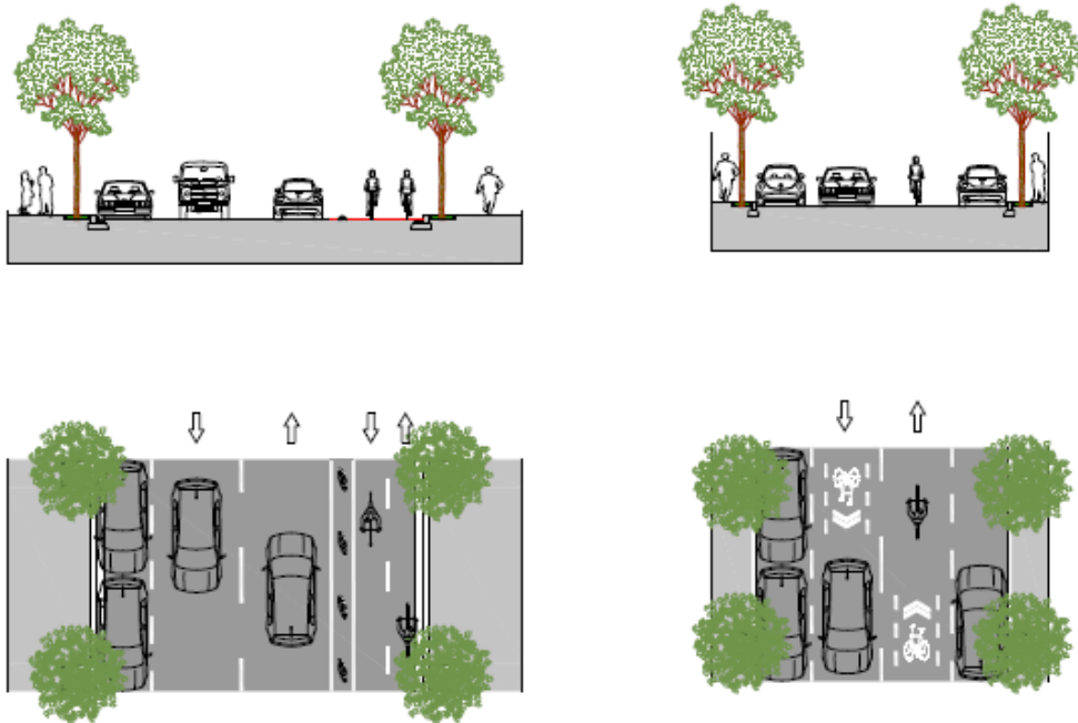
Figura 42. Exemples de seccions de xarxa segregada i xarxa compartida
