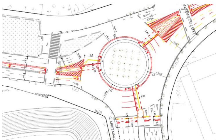
Figura 47.Exemple de configuració de carril bicicletes anul·lar (interior)
