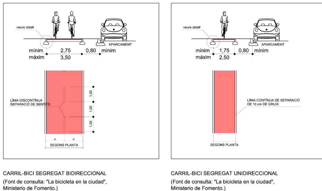
Figura 43. Dimensionament mínim per carrils bicicleta
