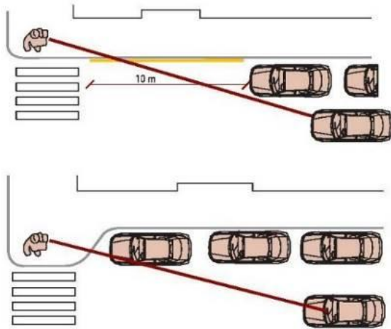
Figura 33. Aplicació de mesures de millora de la visibilitat
