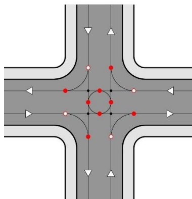
Figura 22.Punts de conflicte en una intersecció en X de doble sentit circulatori
