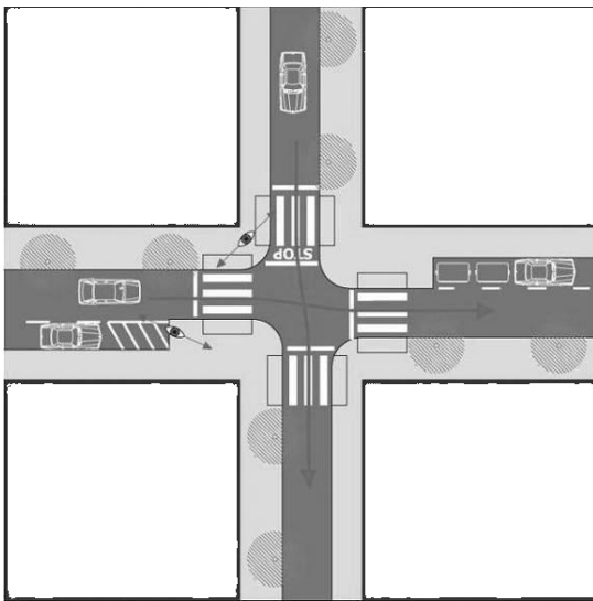
Figura 18. Aplicació de reductors horitzontals de velocitat a carrers d'entre 8 i 10 m
