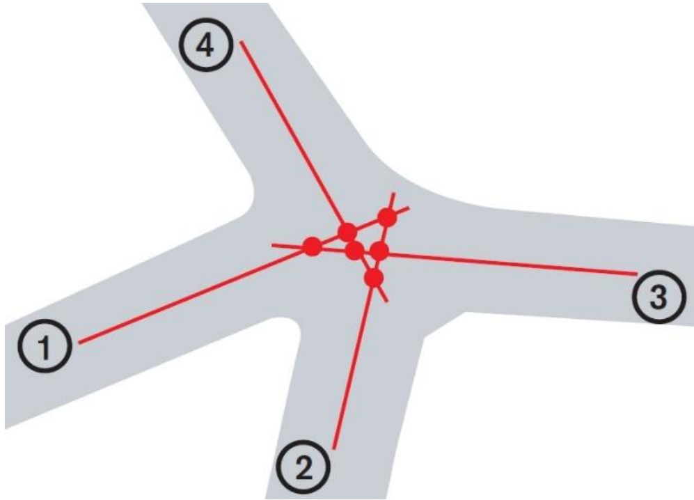
Figura 48. Alineació dels eixos confluent a la rotonda
