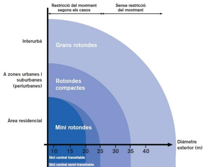
Figura 49. Dimensionament de les rotondes
