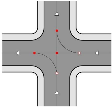
Figura 24. Punts de conflicte en una intersecció en X de sentit únic circulatori
