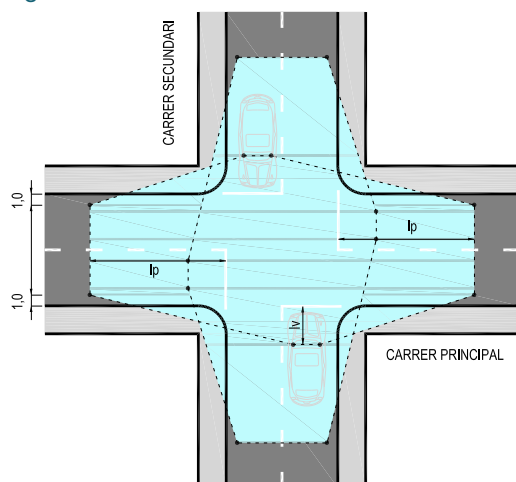
Figura 26. Àrea de visibilitat en interseccions en X
